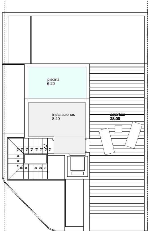
PLANTA CUBIERTA E: 1/75
