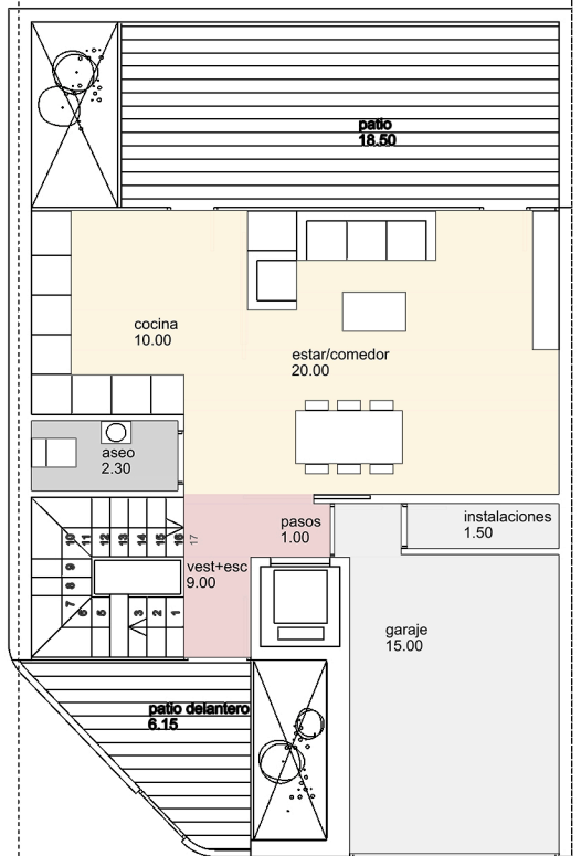
PLANTA BAJA E: 1/75
